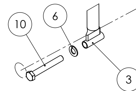
DETALHE C ESCALA 1 : 5
