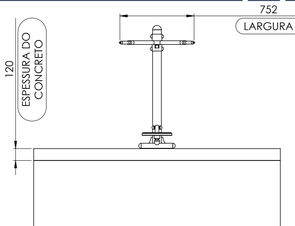
BANCO SERA FIXADO COM PARABOLTS 3/8" X 2 1/2".
