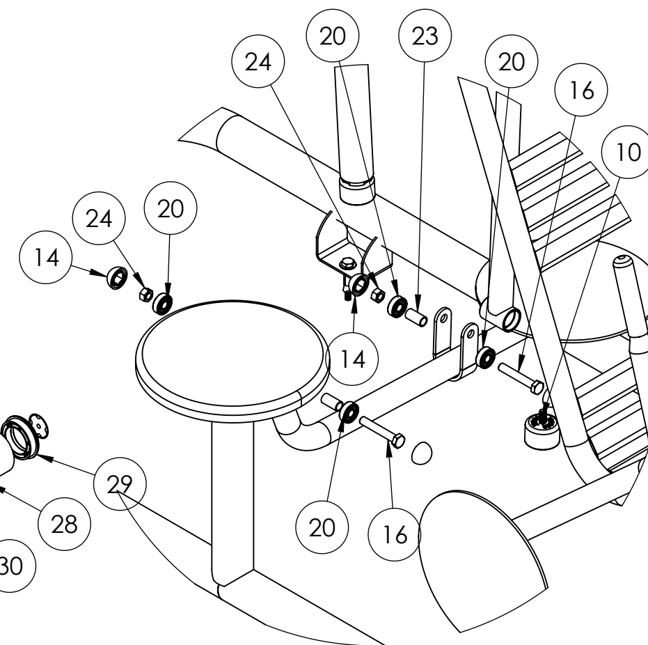
DETALHE D ESCALA 1 : 8
