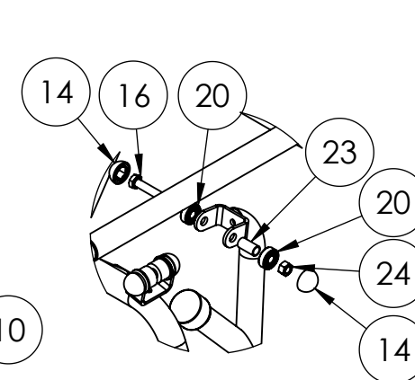
DETALHE E ESCALA 1 : 10
